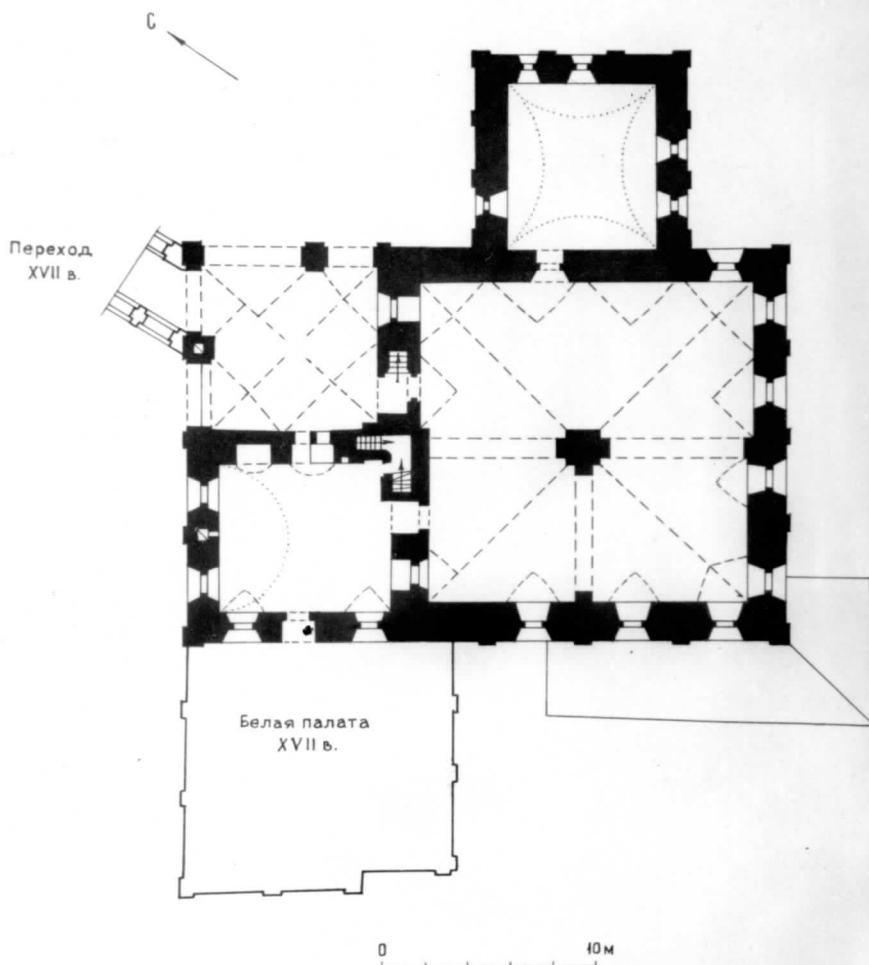
План II-го этажа
